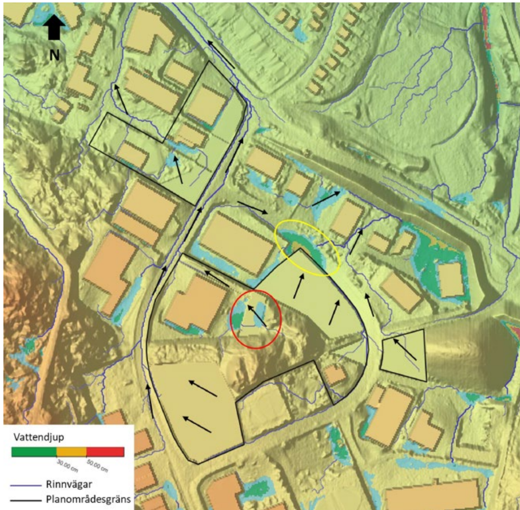
Figur 9: Figuren visar översvämningssituationen vid anpassad höjdsättning inom rödringat område.
