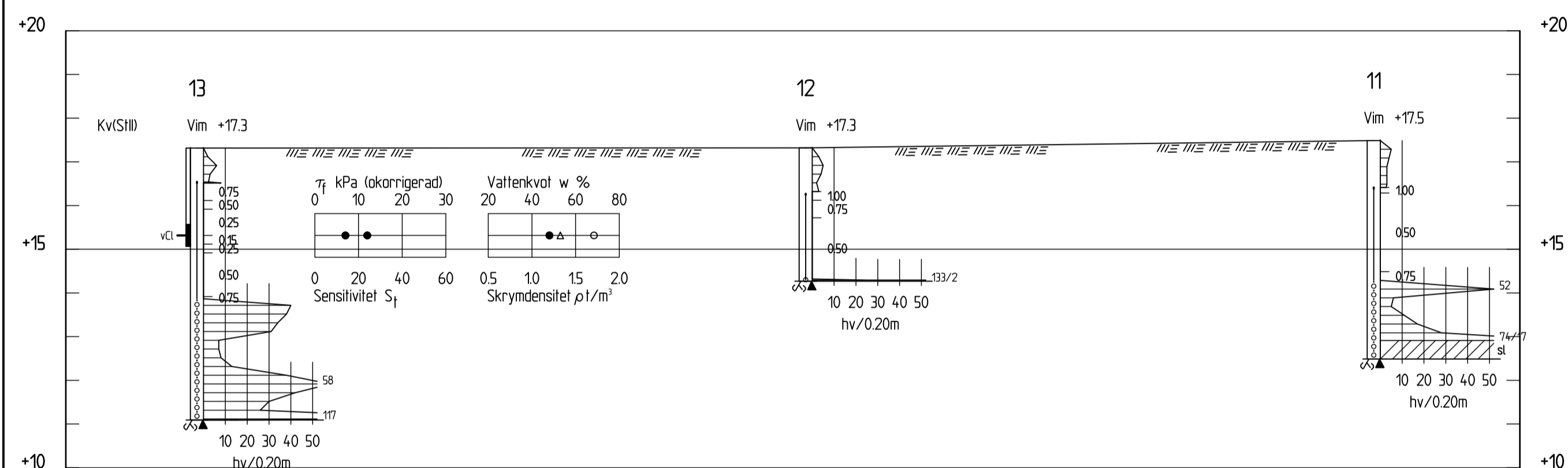
SEKTION A-A 1:100
