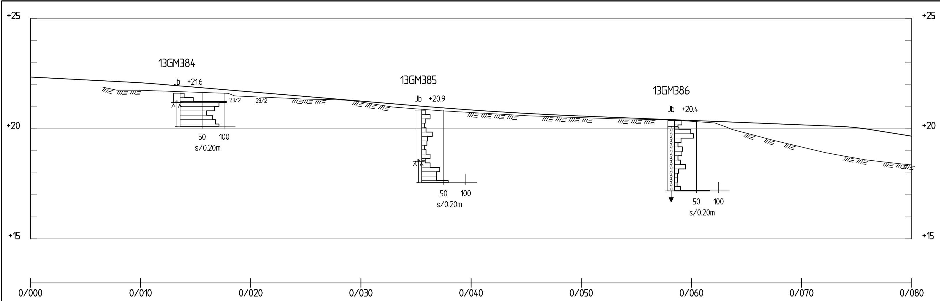
RUDSJÖKROKEN H 1:100 L 1:200
