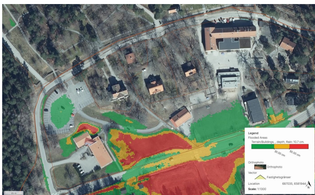
Figur 11: Skyfallsanalys i Scalgo live vid ett 107-mm regn. Bildkälla: Scalgo live.
