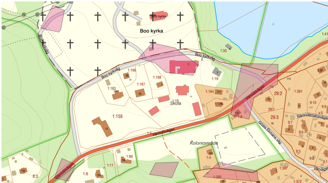
Figur 9: Förutsättningar för skred i finkornig jordart. Rosa område visar aktsamhetsområde för skred i finkornig jordart. Bildkälla: SGUs Förutsättningar för skred i finkornig jordart
