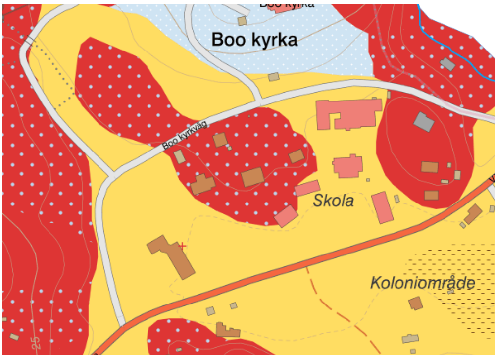
Figur 8: Övergripande jordartskartering. Rött utgörs av berg, gult utgör postglacial lera och ljusblå prickar utgör tunt moränlager. Bildkälla: SGUs jordartskartering.
