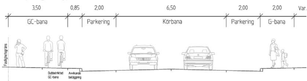
Sektion som visar disponering av Ektorpsvägens gaturum efter ombyggnad. Måtten är angivna i meter.
