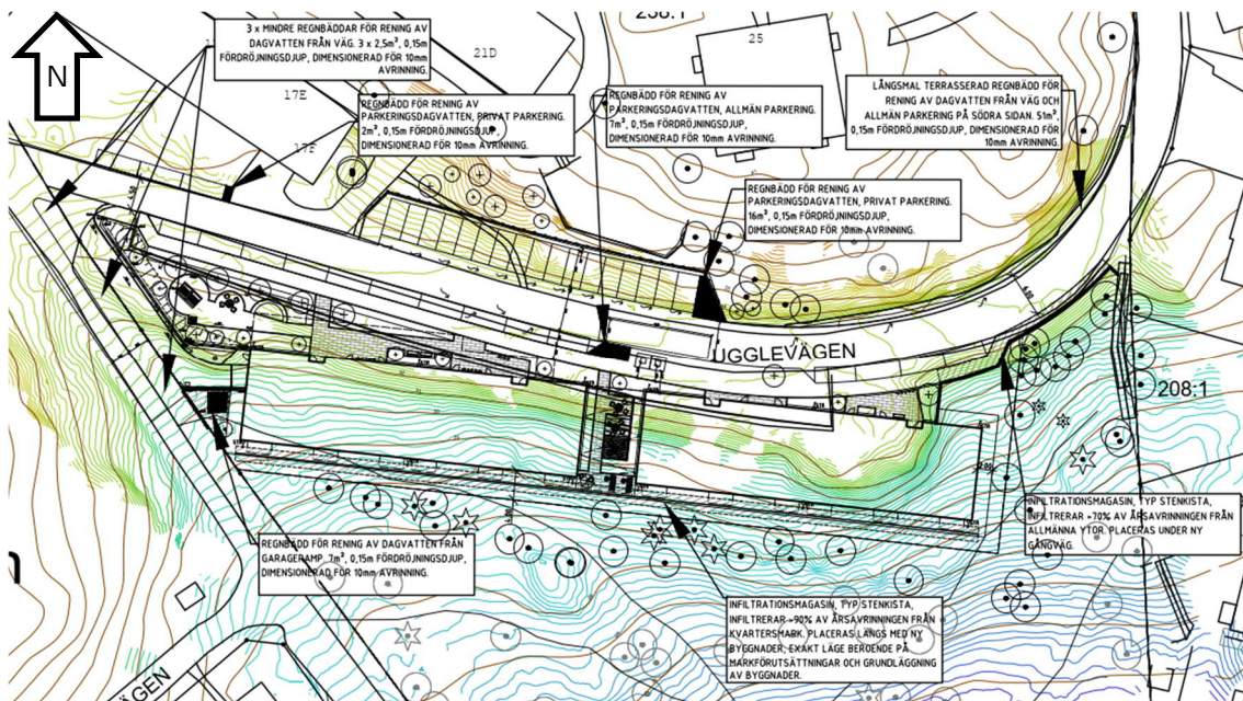
Figur 6. Föreslagen dagvattenhantering.
