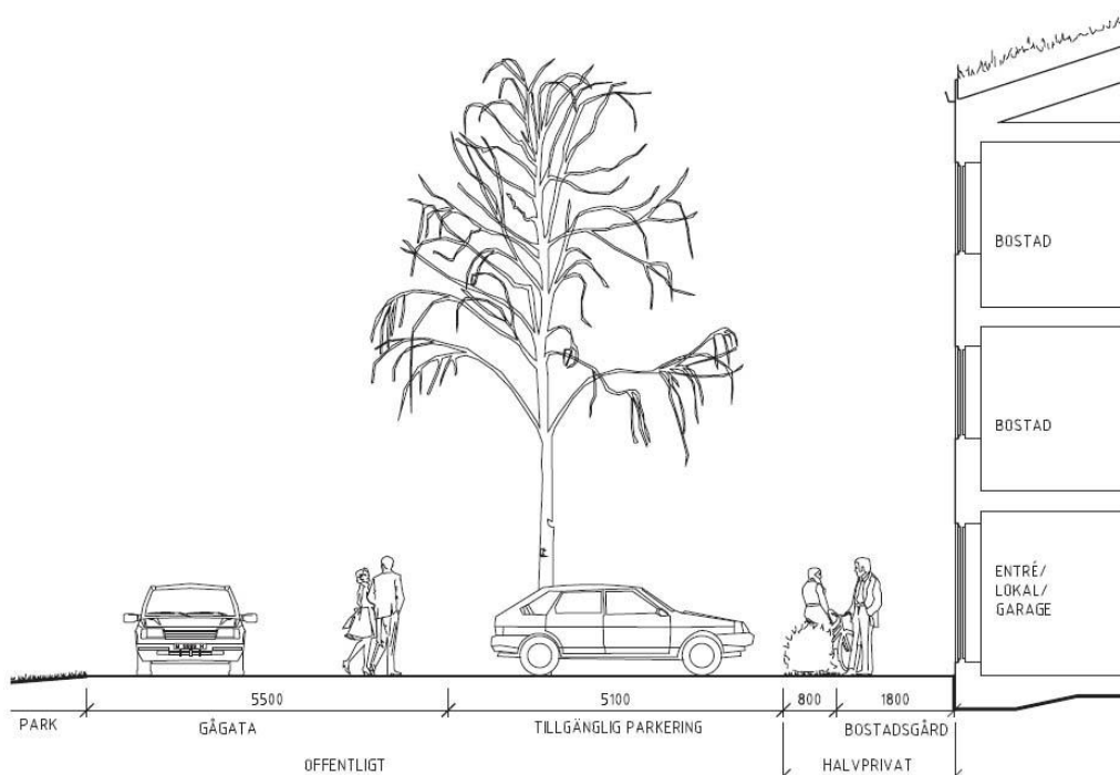
Principsektion genom gångfartsgata-tvärställd parkering och förgårdsmark till bostadsbus.
