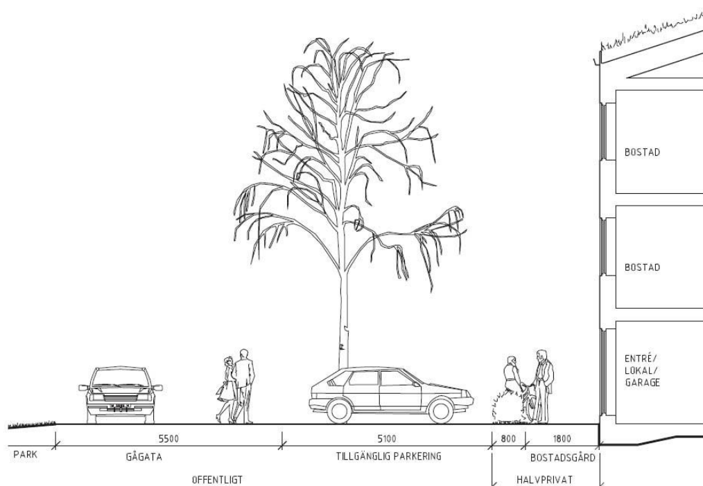
Principsektion genom gångfartsgata-tvårvårdad parkering och förgårdsmark till bostadsbus.
