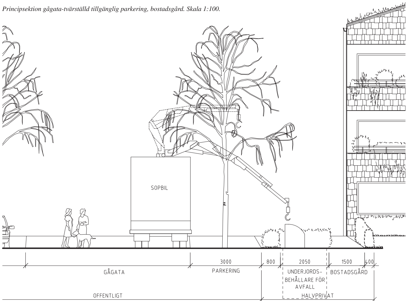
Principsektion gågata-sopbil-avfallskäril-bostadsgård. Skala 1:100.
