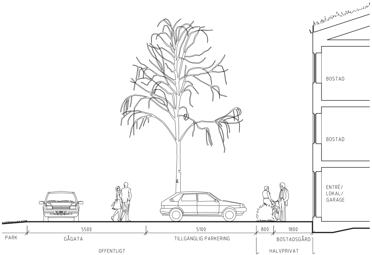
Principsektion gågata-tvärställd tillgänglig parkering, bostadsgård. Skala 1:100.
