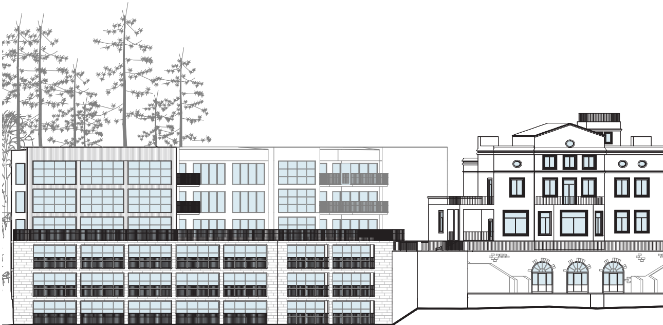
Fasad mot söder (Baggensfjärden), skala 1:400.
