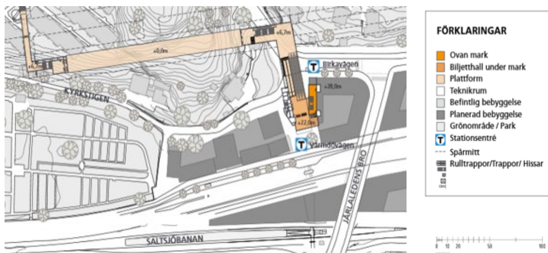
Figur 7. Situationsplan för kommande tunnelbana vid Saltsjö Järsla, mellan planrådets östra och västra kvarter. De två tunnelbaneentréerna är markerade med T. Tidigare förslag på strukturskiss. Illustration: Sweco.
