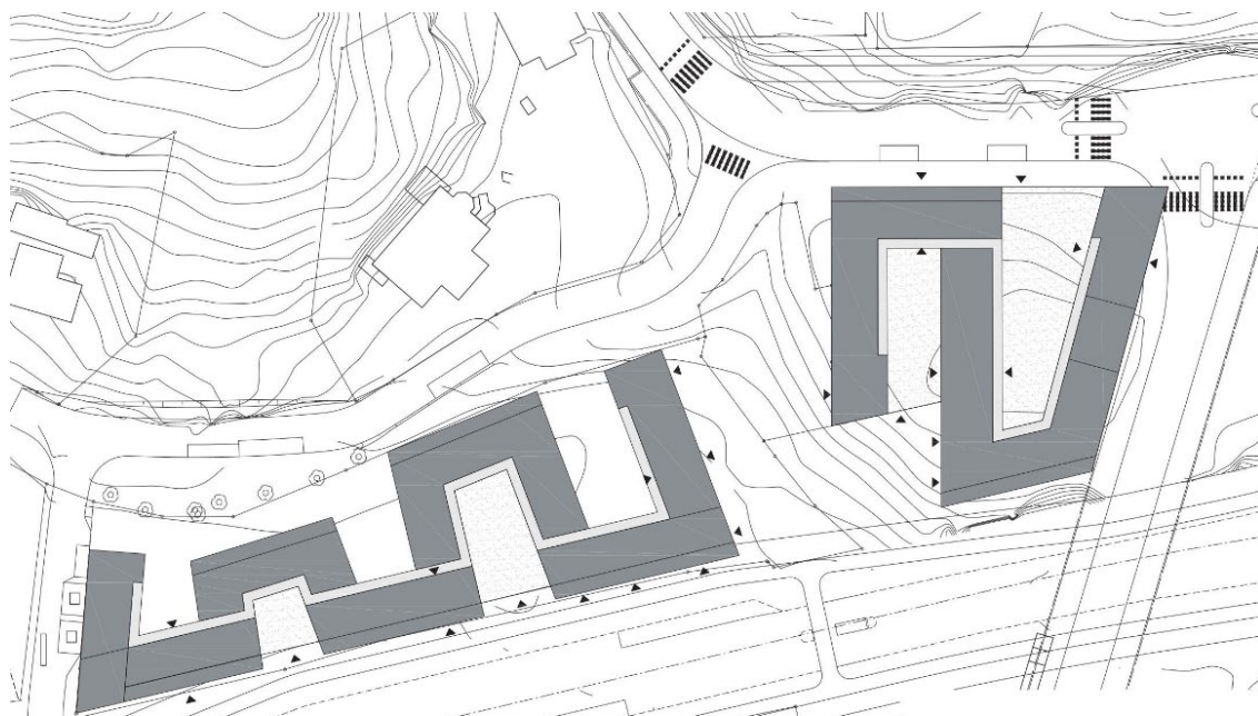
Figur 3. Situationsplan utkast 2019-10-04. Av: Semrén & Månsson arkitekter, ALM Equity.
