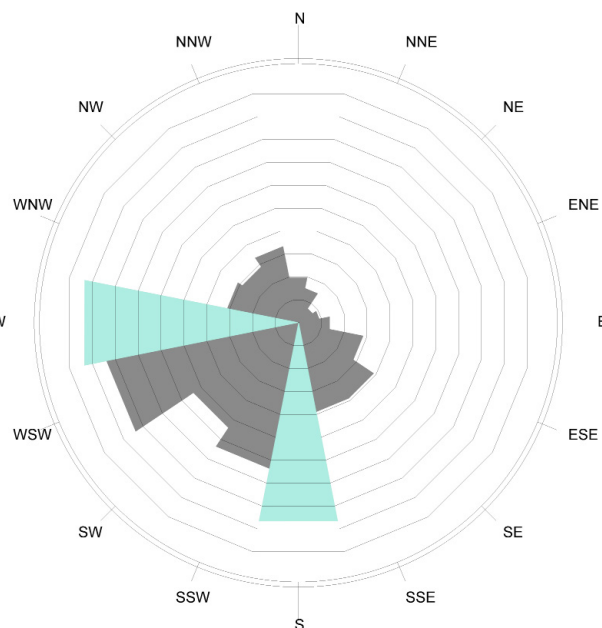
Figur 9: Årlig distribution av vindriktningar vid Bromma flygplats. De simulerade vindriktningarna är färgade med ljusblått. Varje cirkel i diagrammet motsvarar här 21 timmar.
