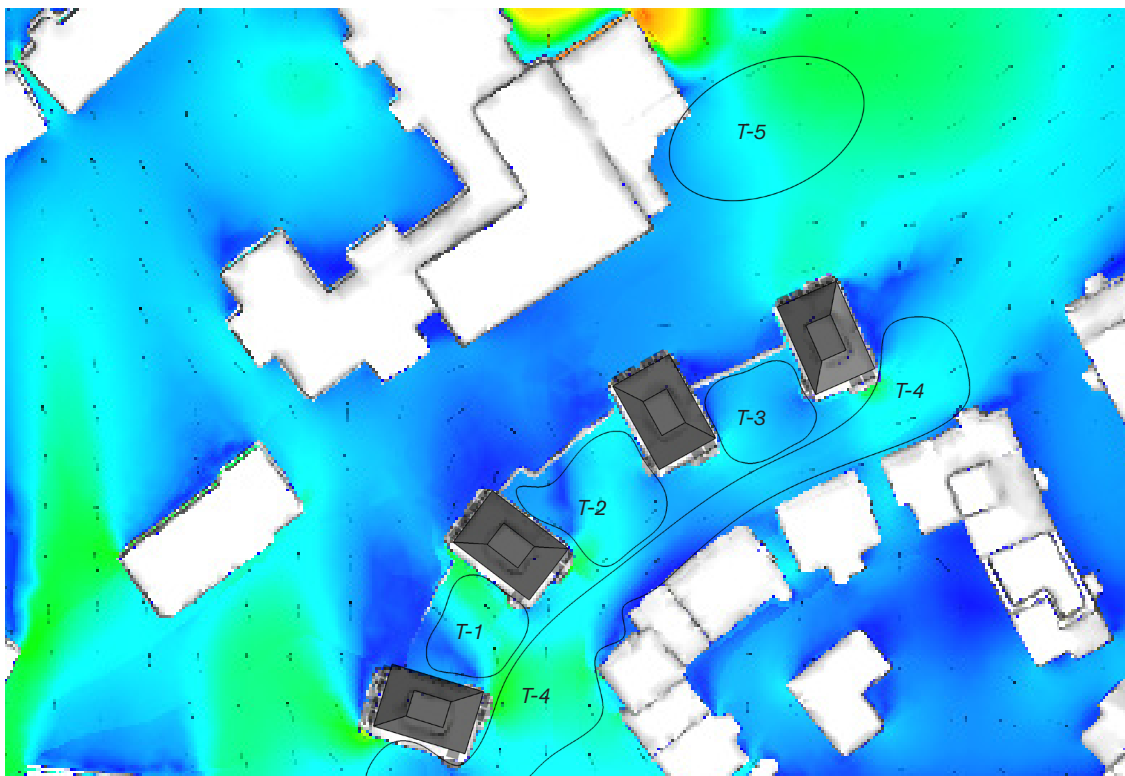
Figur 11: Vindhastigheten simulerad 1,5 meter från marken (Vind från syd med hastigheten 5 m/s)
