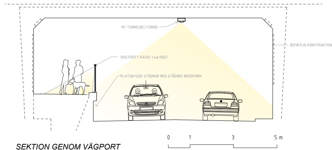
SEKTION GENOM VÄGPORT
