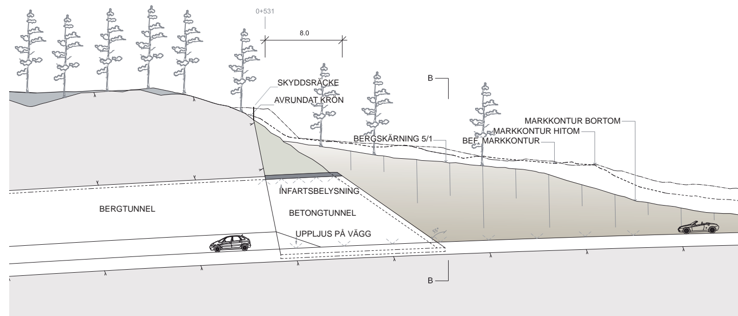
ILLUSTRATIONSSEKTION PÅ SÖDRA TUNNELMYNNINGEN
