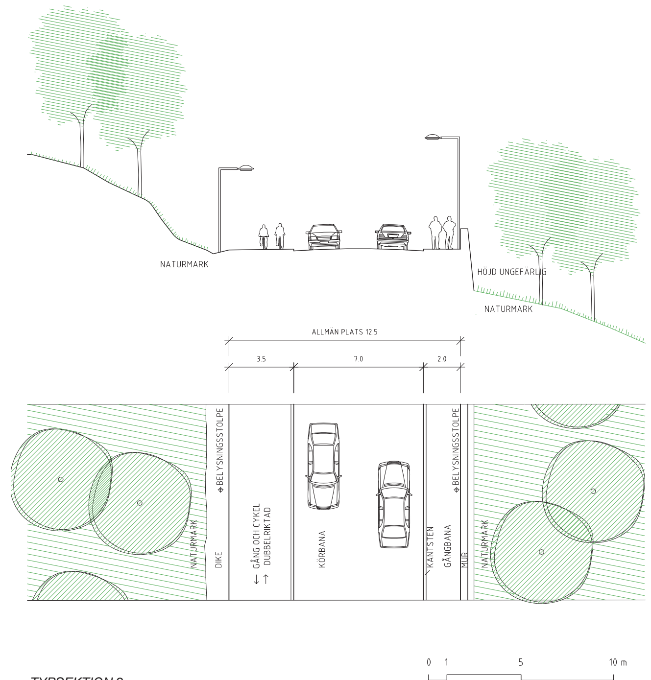
TYPSEKTION 2
