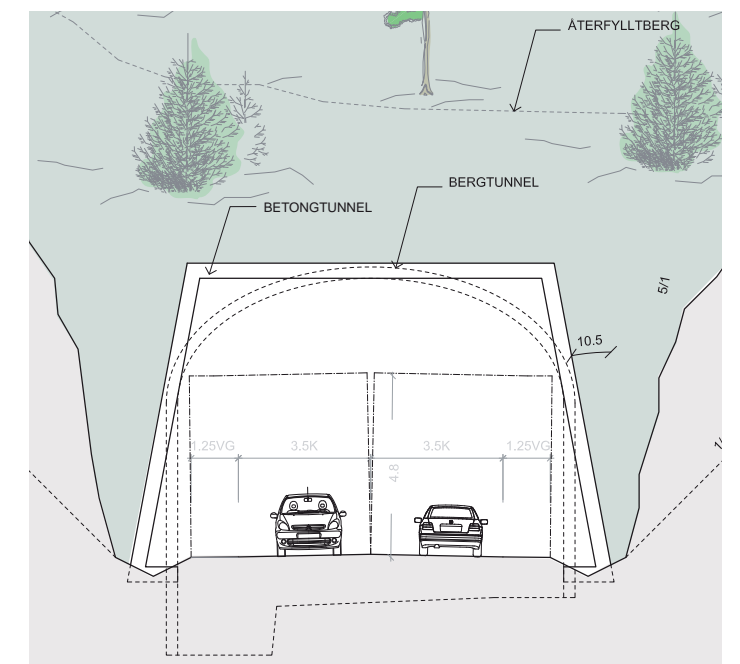
SEKTION B
