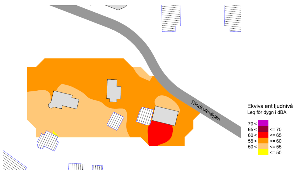
Bostäder, Tändkulevägen. Ekvivalent ljudnivå vid fasad, frifältsvärde. Bild: ÅF
