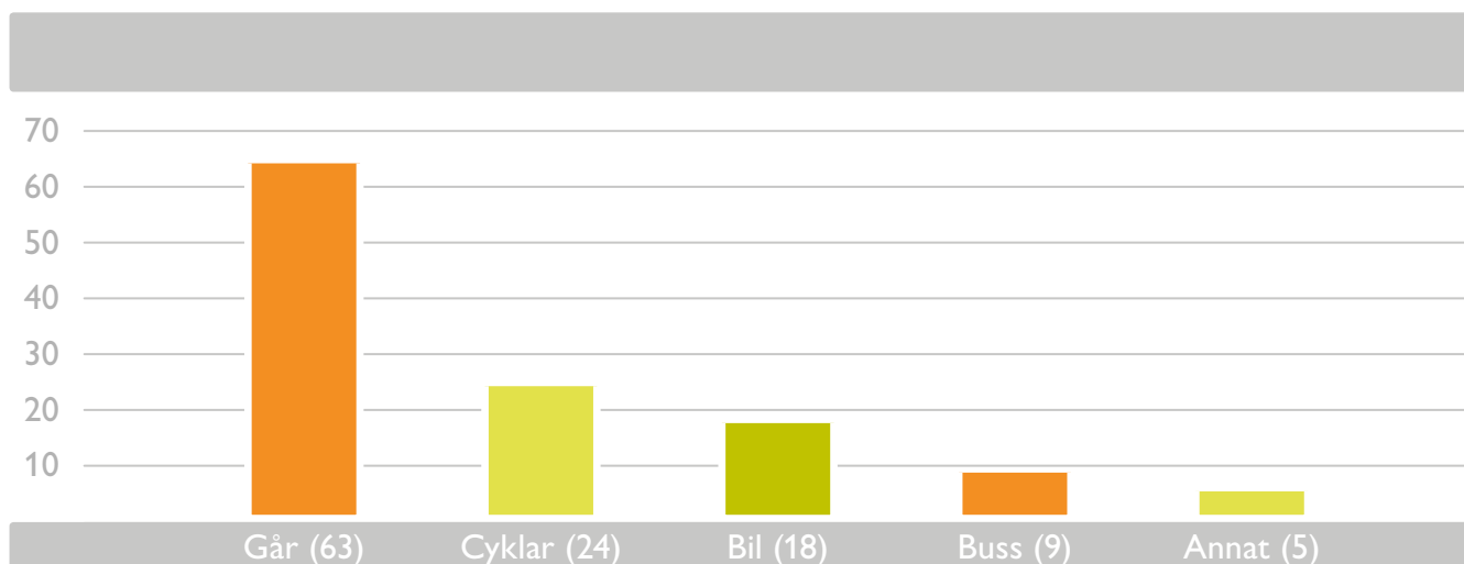
Figur 3: Transportmedel (flervalfråga).
