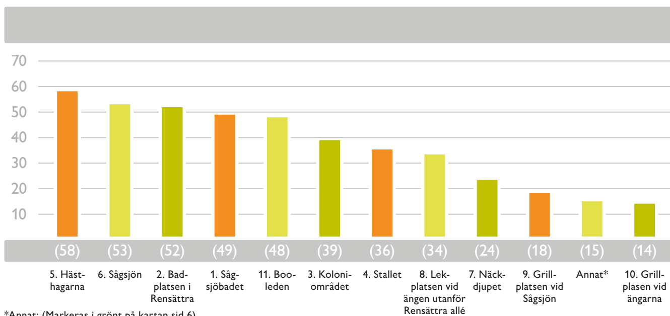
Figur 5. Favoritplatser.
