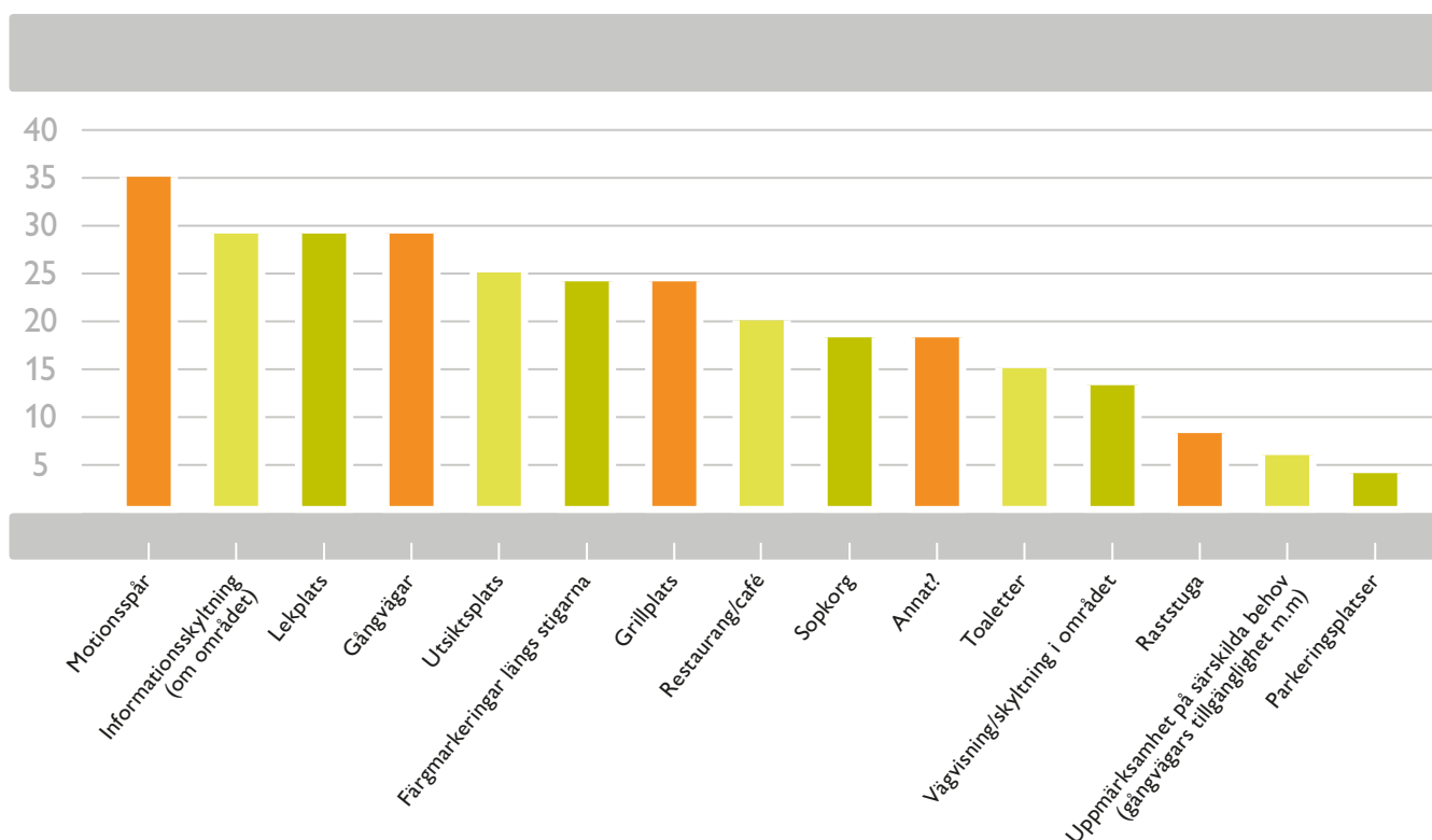
Figur 10. Önskade servicefunktioner.
