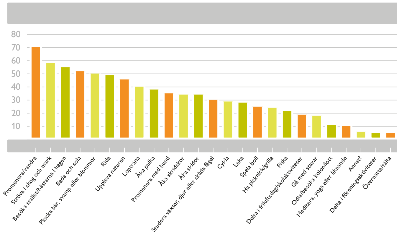
Figur 11. Önskade aktiviteter.
