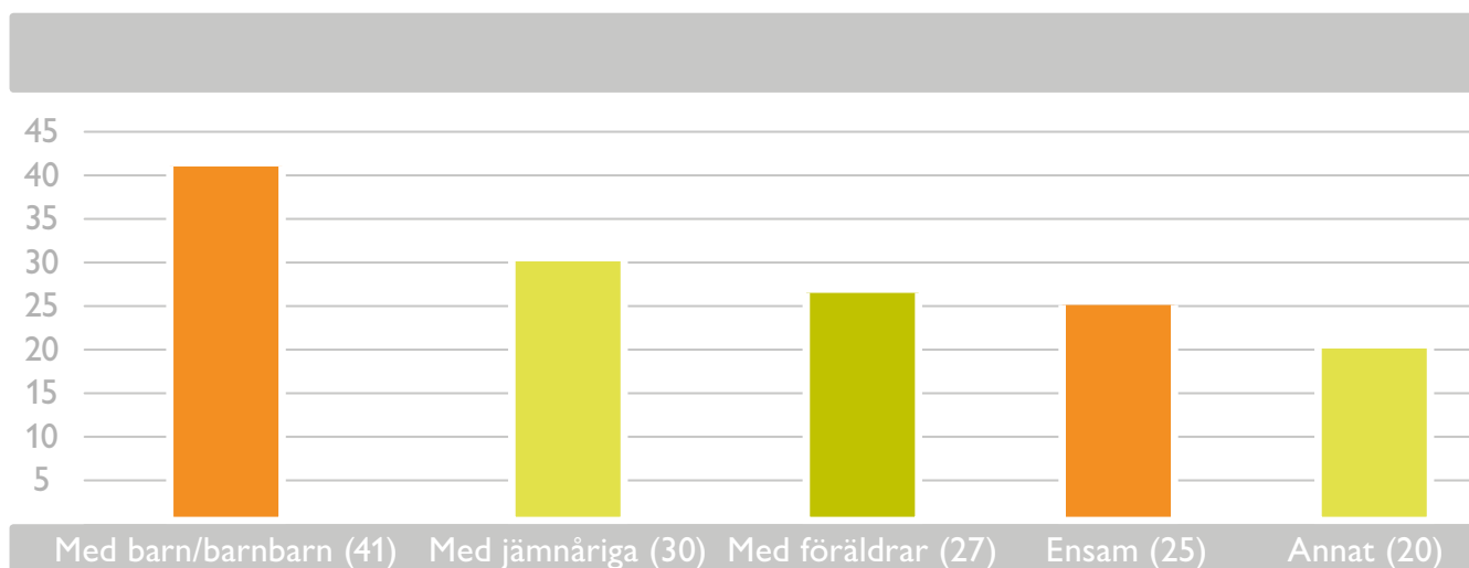
Figur 4. Besöksällskap (flervalsfråga).
