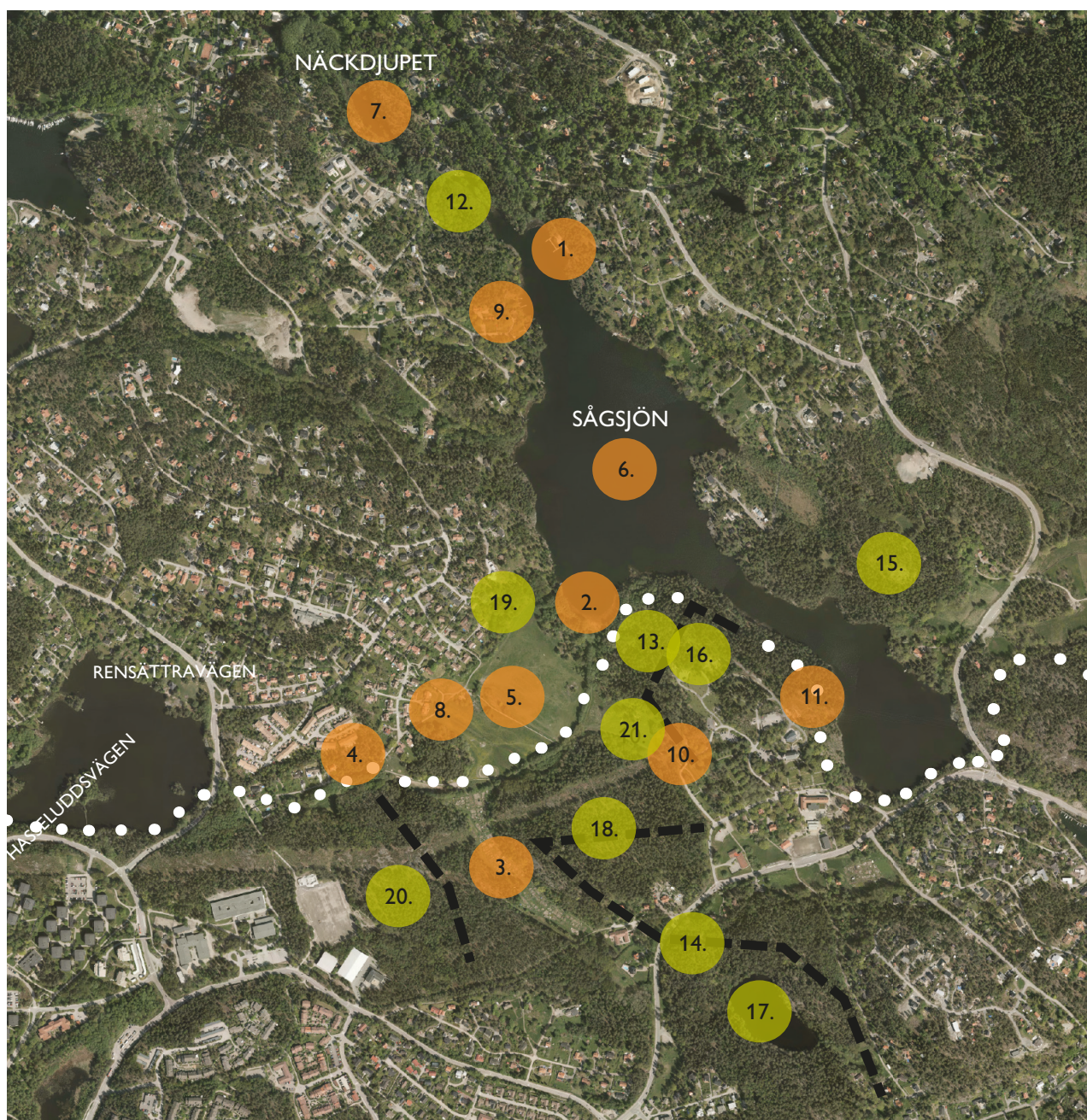
Figur 6 Målpunkter.
