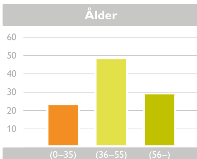
Figur 1: Demografisk översikt.
