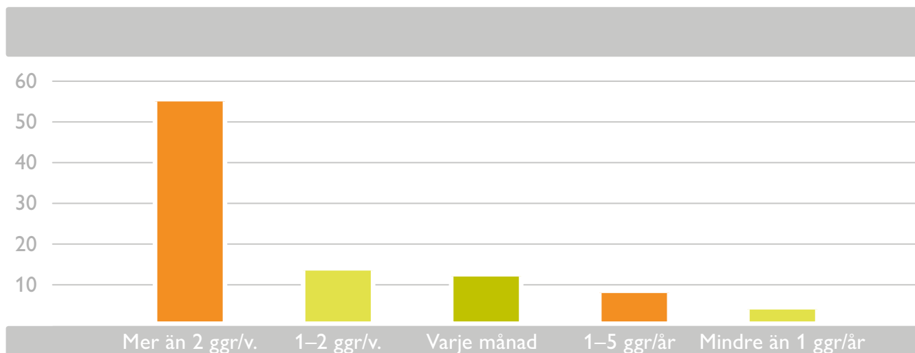
Figur 2: Besöksfrekvens.
