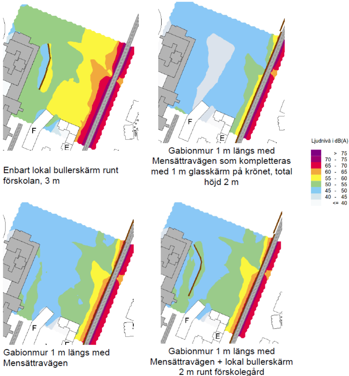
Figur 4. Beräkningar med bullerskärmar (ekvivalent ljudnivå 1,5 m över mark i dB(A). Avser dagvärde kl 06-18).
