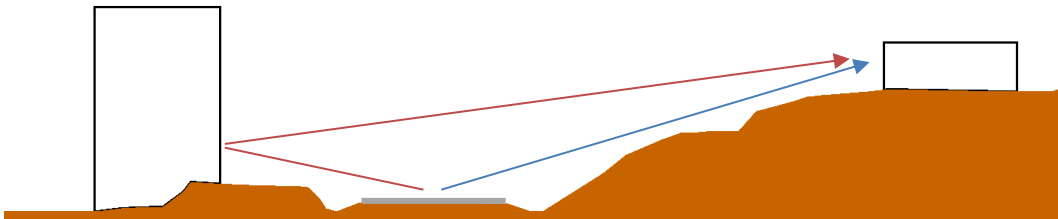
Figur 6. Sektion kring Mensättravägen, med planerad (vänster) och befintlig bebyggelse (höger). Blå pil avser direktljud och röd pil avser reflekterat ljud.
