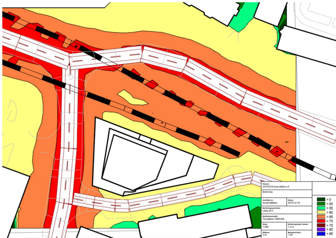
Ekvivalent (L Aeq dBA) ljudnivå 1,5 meter ovan mark .
