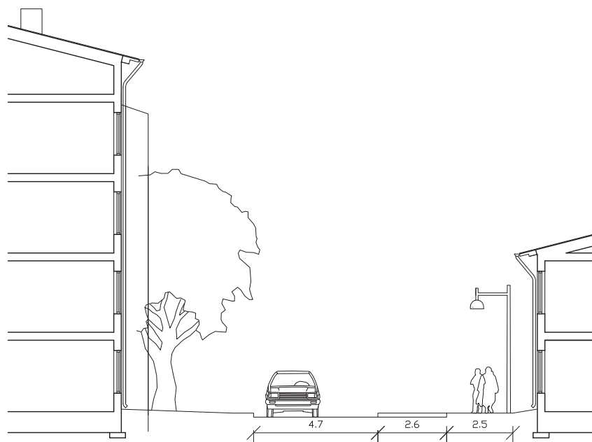
SEKTION KOMMUNAL GATA MELLAN FLERBOSTADSHUS OCH FÖRSKOLA
