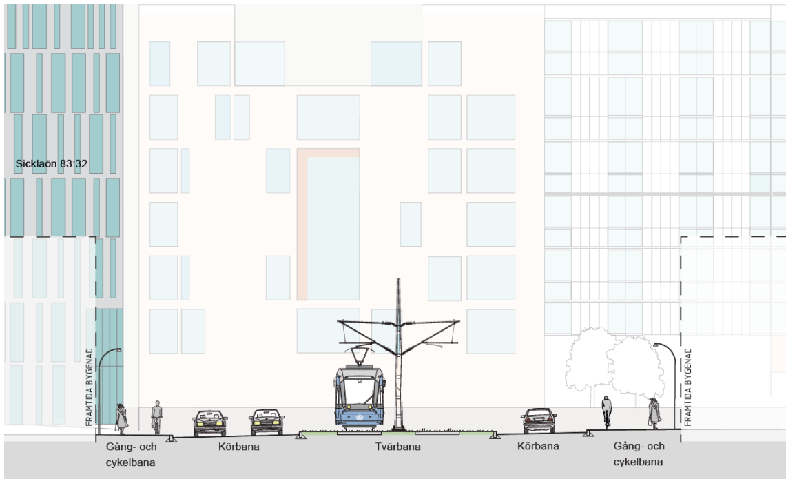
Sektion 1. Utformning av södra Uddvägen, vy mot Sicklavägen. GRID Arkitektur AB
