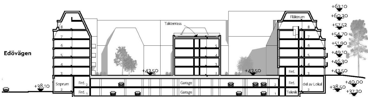
Principsektion, vy från väst, kvarter Hantverkarshuset
