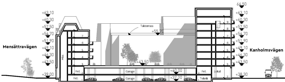
Principsektion, vy från norr, kvarter Hantverkarshuset
