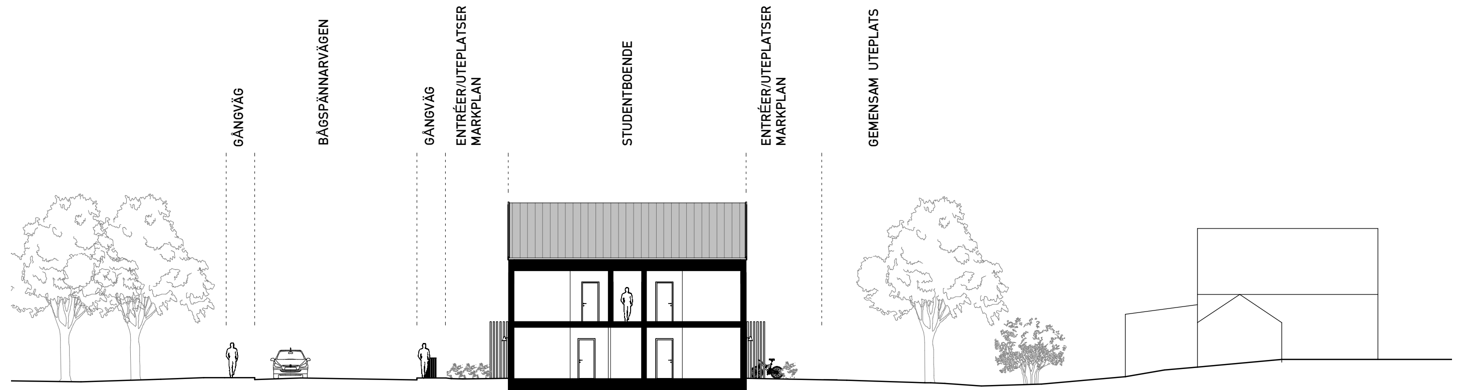
SEKTION B-B BÅGSPÄNNARVÄGEN
