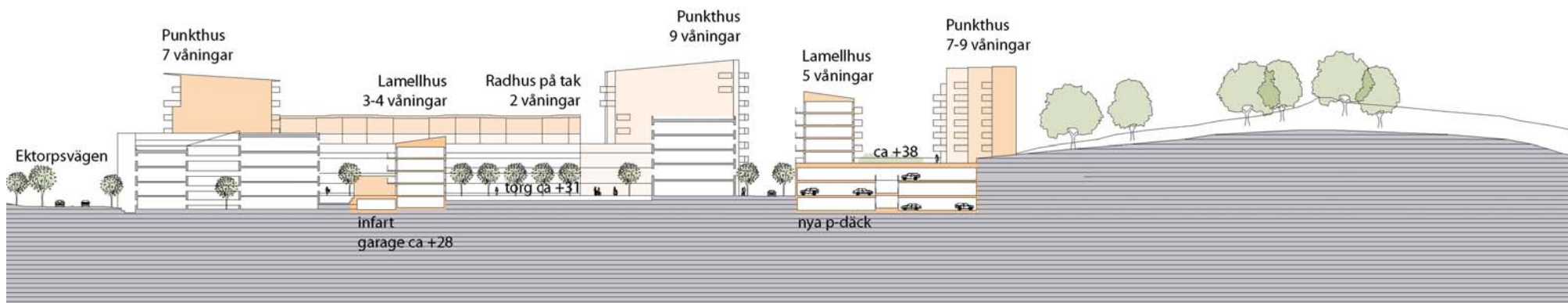
Sektion mot norr
