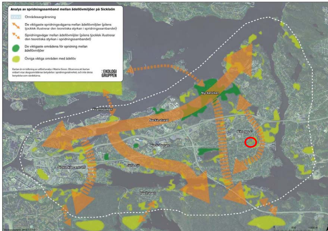
Spridningsanalys Sicklaön, Ekologigruppen 2014. Planområdet markerat med röd ring.
