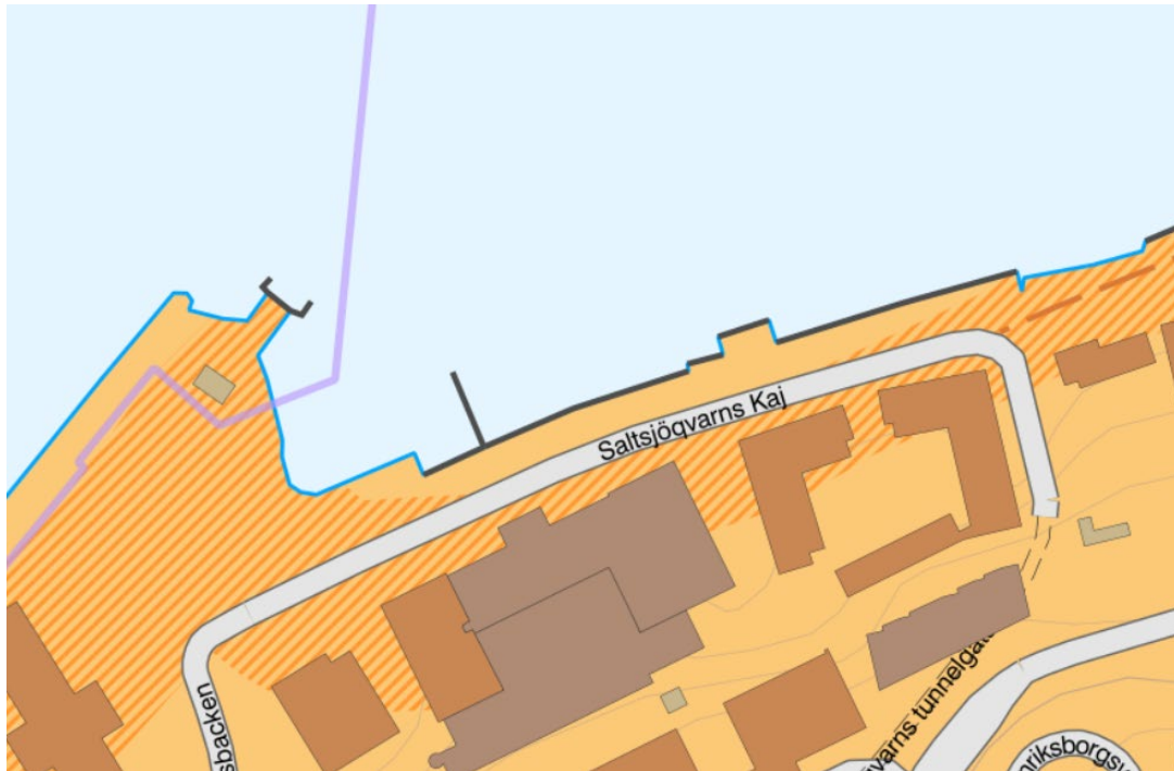
Figur 4. Rödskräfferad markering visar lera och silt. Generell skredrisk inom aktsamhetsområde. Underlag SGU:s skredriskkarta, 2025.
