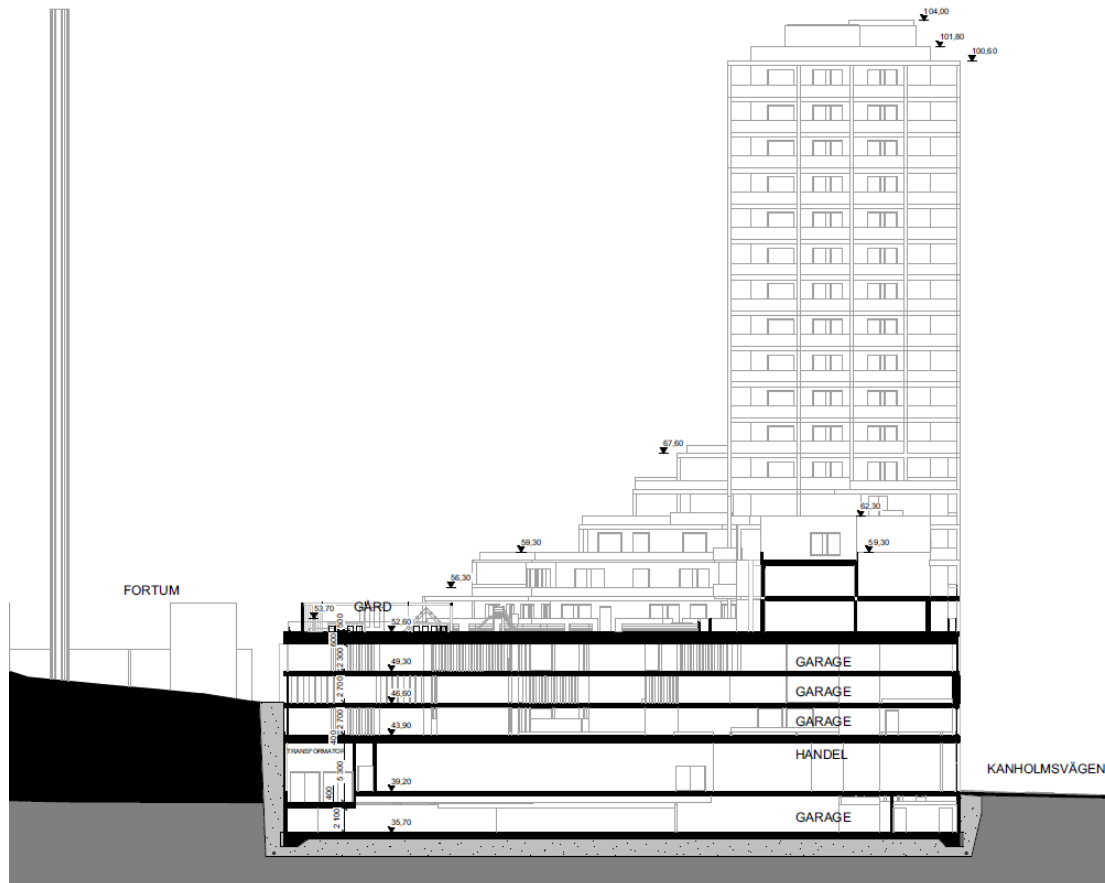
Sektion, Kvarter Parkeringshuset och intilliggande panncentral, vy från söder
