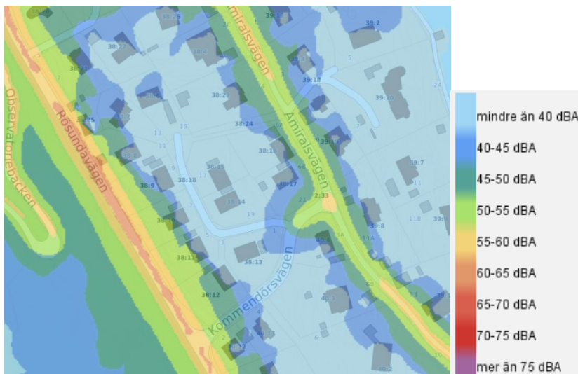
Figur 8. Ekvivalenta bullernivåer från vägtrafik.
