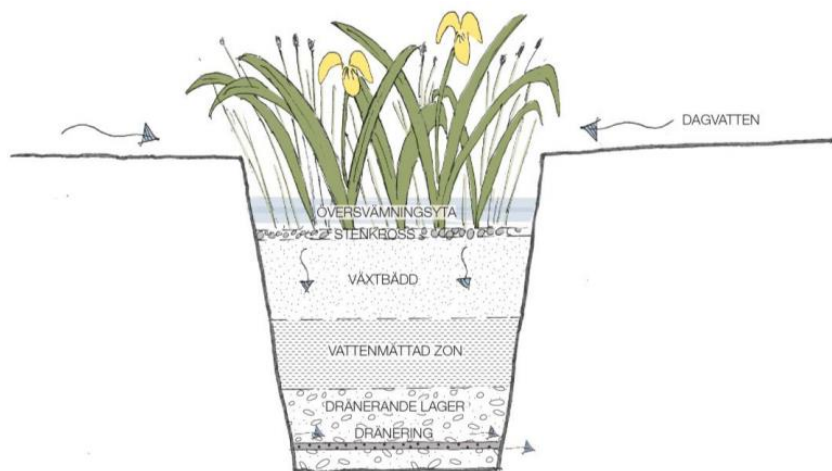
Figur 18. Exempel på växtbäddsutformning för att rena dagvattnet. Illustrationen kommer från dagvattenutredningen, Norconsult.
