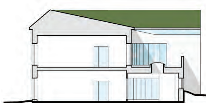
Sektion B-B
