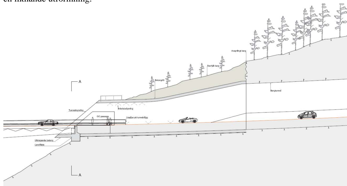
Utformning av tunnelmynning.
