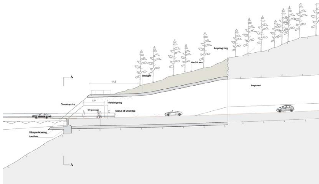
Utformning av tunnelmynning.
