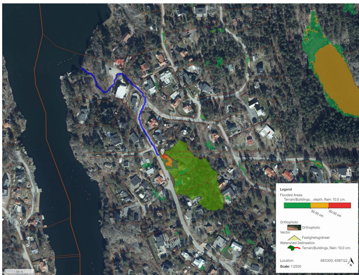
Figur 10. Skyfallsanalys i Scalgo live vid ett 107-mm regn.
