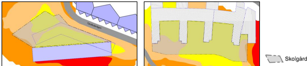
Dygnskvivalent ljudnivå vid förskola/förskolegård samt skolgård söder om hus 9. Bilder: ÅF
