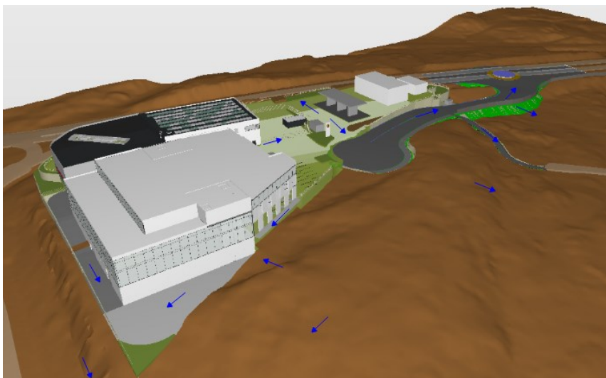
Figur 52: Skyfallsavrinning efter planerad exploatering, sett från sydöst.
