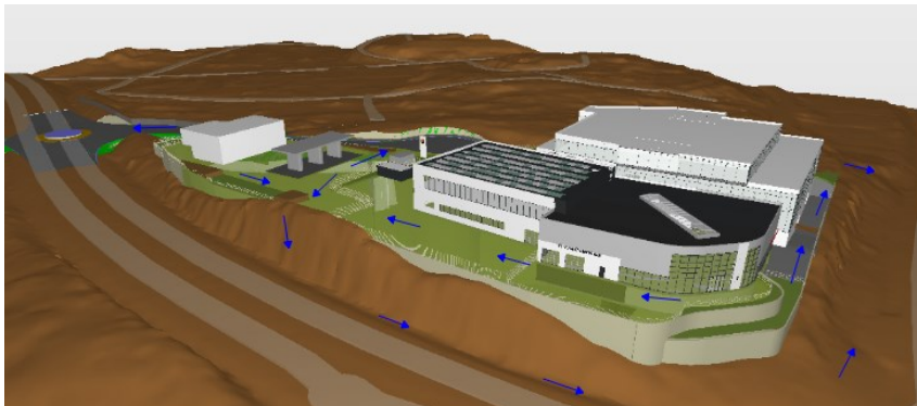
Figur 51: Skyfallsavrinning efter planerad exploatering, sett från sydväst.
