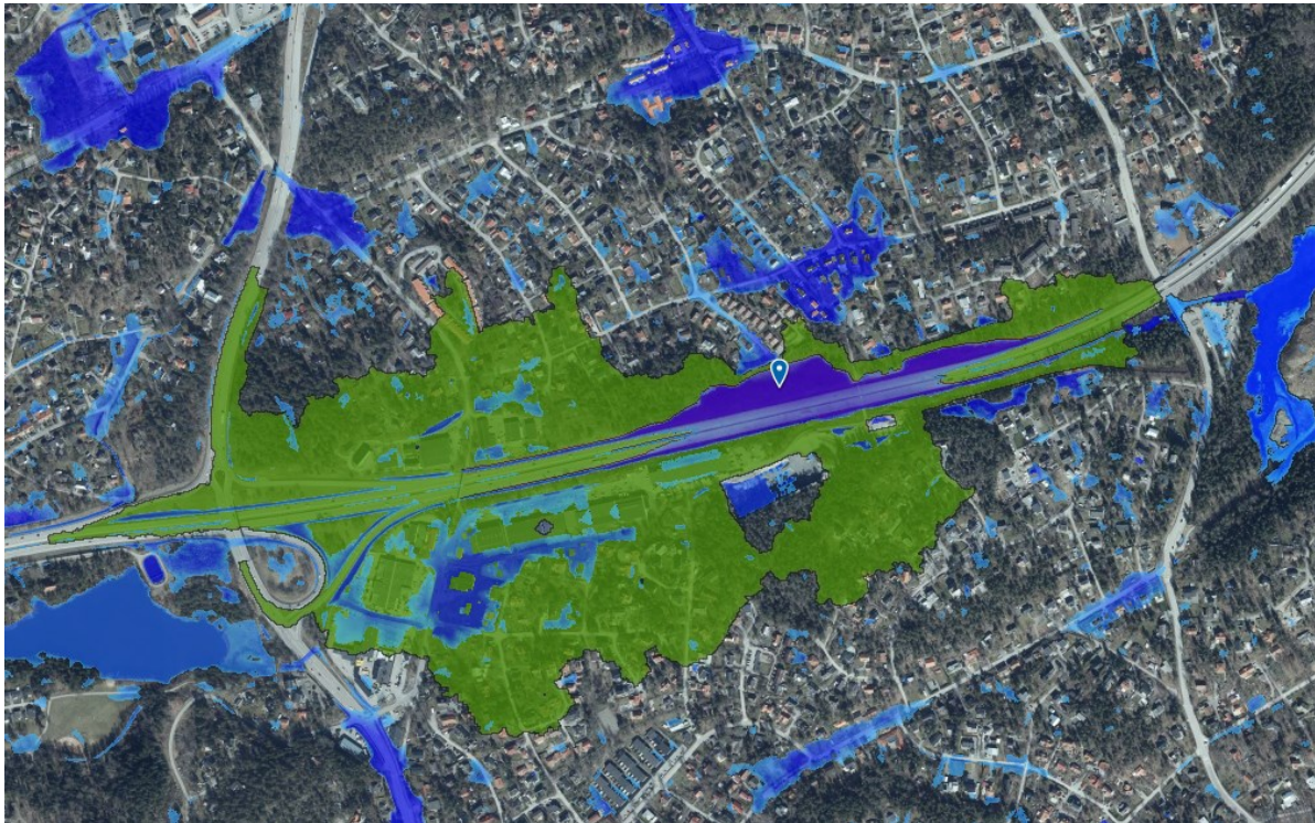
Figur 45: Lågpunkt på Värmdöleden (Scalgo Live 2023-10-09).
