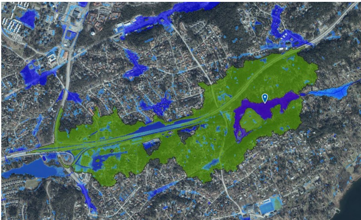
Figur 48: Andra lågpunkten längs avrinningsvägen mot Baggensfjärden (Scalgo Live 2023-10-09).
