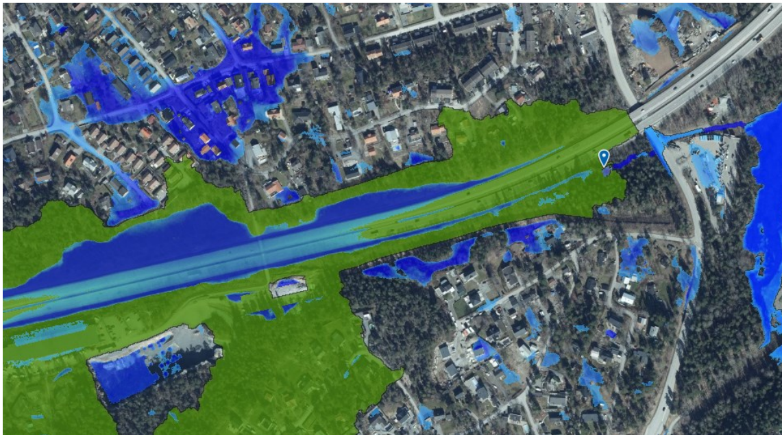
Figur 47: Placering höjdrygg (Scalgo Live 2023-10-09).
