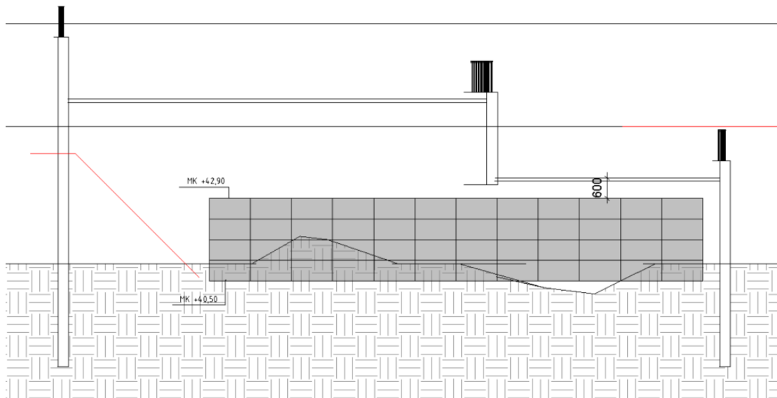
Figur 29: Tvärsnitt kassettmagasin i nord.
