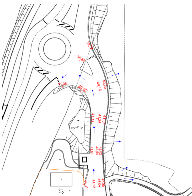
Figur 50: Skyfallsavrinning kommunal väg
