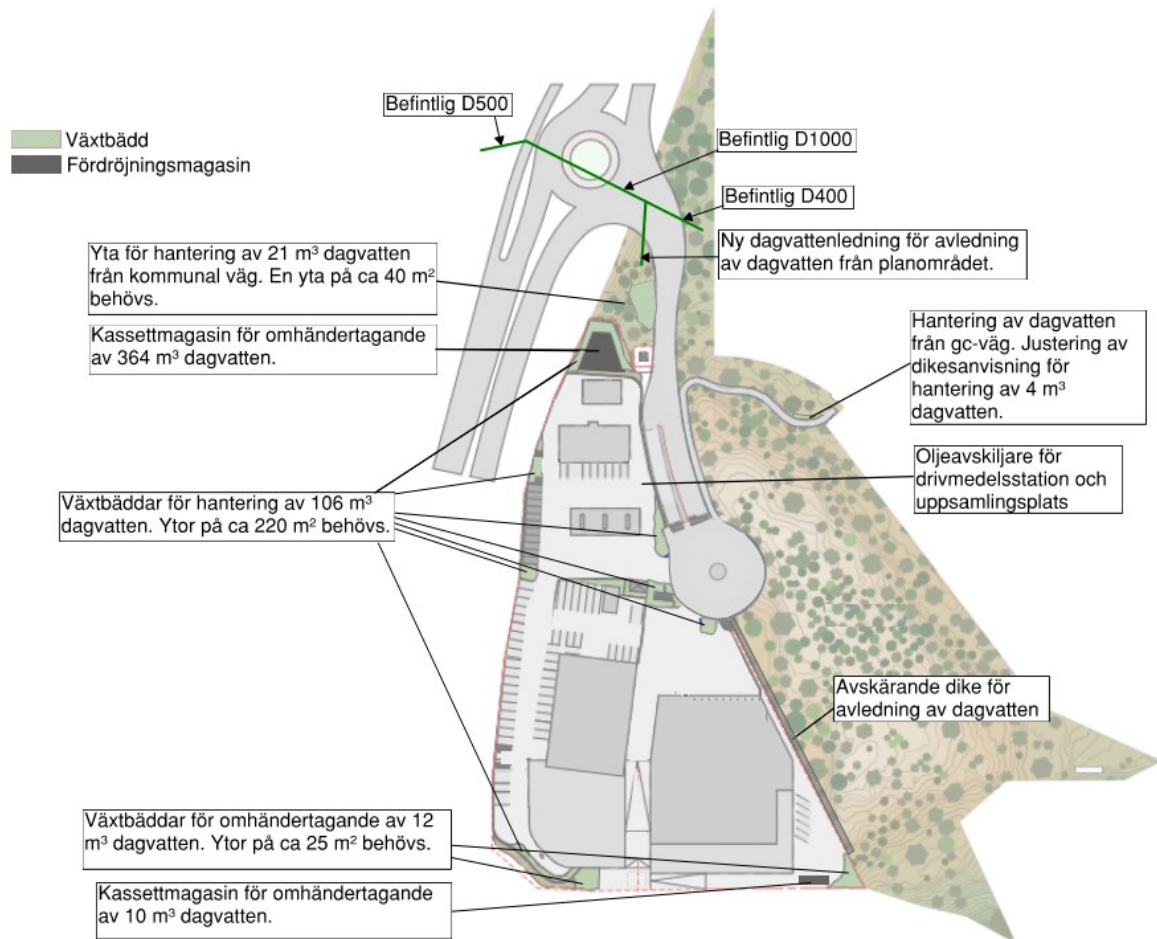
Figur 34: Förslag på åtgärder.
