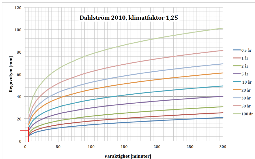
Figur 25: Nederbördsvolym som funktion av varaktighet och återkomsttid (Svenskt vatten P110).
