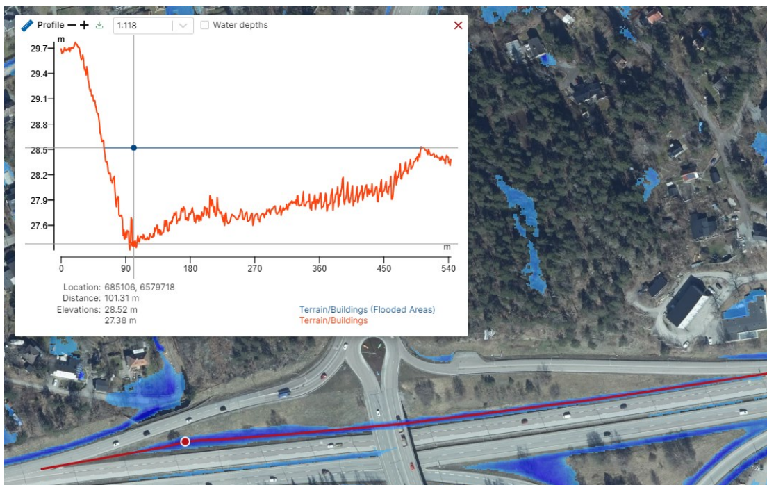
Figur 8: Avrinningsväg i befintligt dike söder om planområdet (Scalگو Live 2023-09-02).
