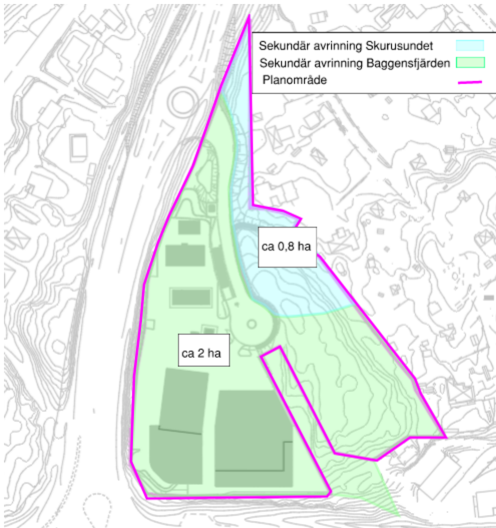
Figur 44: Skyfallsavrinning från planområdet efter planerad exploatering.
