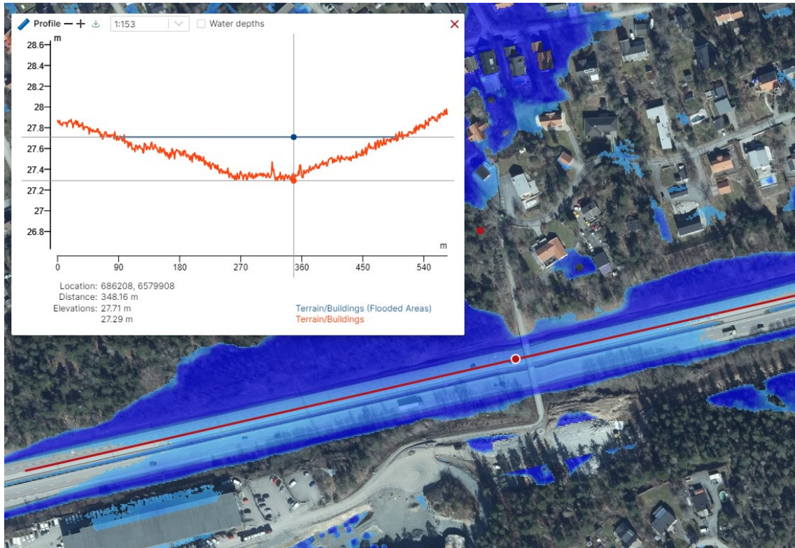
Figur 46: Maximal översvämningsnivå på väg 222 vid skyfall (Scalgo Live 2023-10-09).
