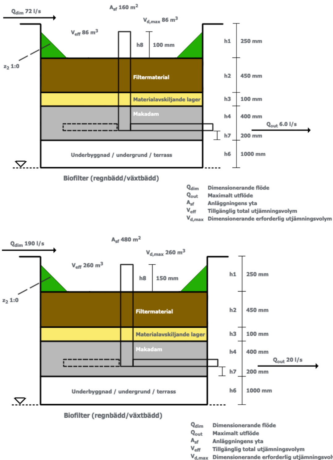
Figur 12. Schematisk profil av växtbädd (enligt Stormtac), med de dimensioner som ligger till grund för beräkningarna för allmän platsmark (ovan) samt kvartersmark (under)
