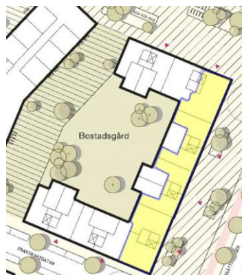
Figur 8. Planlösningen hos gulmarkerade lägenheter behöver bulleranpassas så att minst hälften av bostadsrummen i dessa bostäder ska vara vända mot en sida där 55 dBA ekvivalent ljudnivå inte överskrids vid fasaden.
