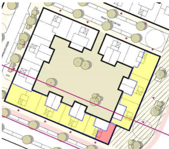
Figur 6. Planlösningen hos gul- och rödmarkerade lägenheter behöver bulleranpassas så att minst hälften av bostadsrummen i dessa bostäder ska vara vända mot en sida där 55 dBA ekvivalent ljudnivå inte överskrids vid fasaden. För den rödmarkerade lägenheten bedöms detta som mycket svårt att uppnå.
