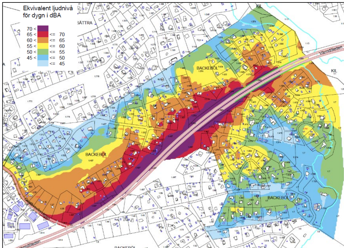
Figur 2. Ekvivalent ljudnivå 5 m över mark (Structor, 2018).
