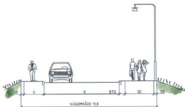
Sektion genom Hedenströmsväg
