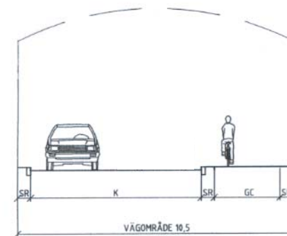
Tollaretunneln sektion
