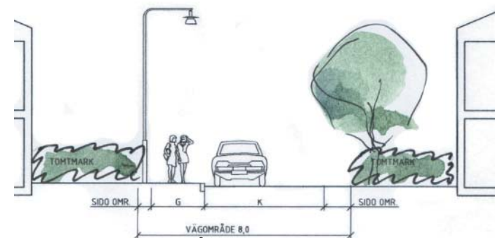
Sektion genom lokalgatan i dalgången
