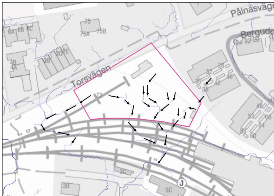
Figur 6. Rinnvägar och avrinningsriktning inom och i direkt anslutning till planområdet. (SCALGO, 2024). Planområdesgräns i magentafärgad linje.
