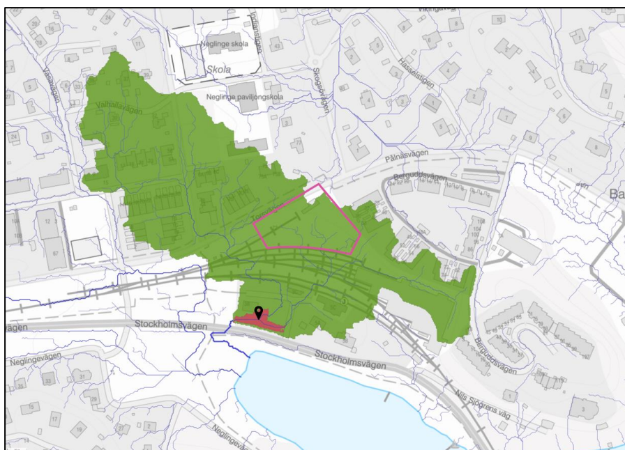
Figur 7. Avrinningsområden uppströms planområdet (SCALGO, 2024). Avrinningsområdet är cirka 5,3 ha stort. Planområdesgräns i magentafärgad linje.
