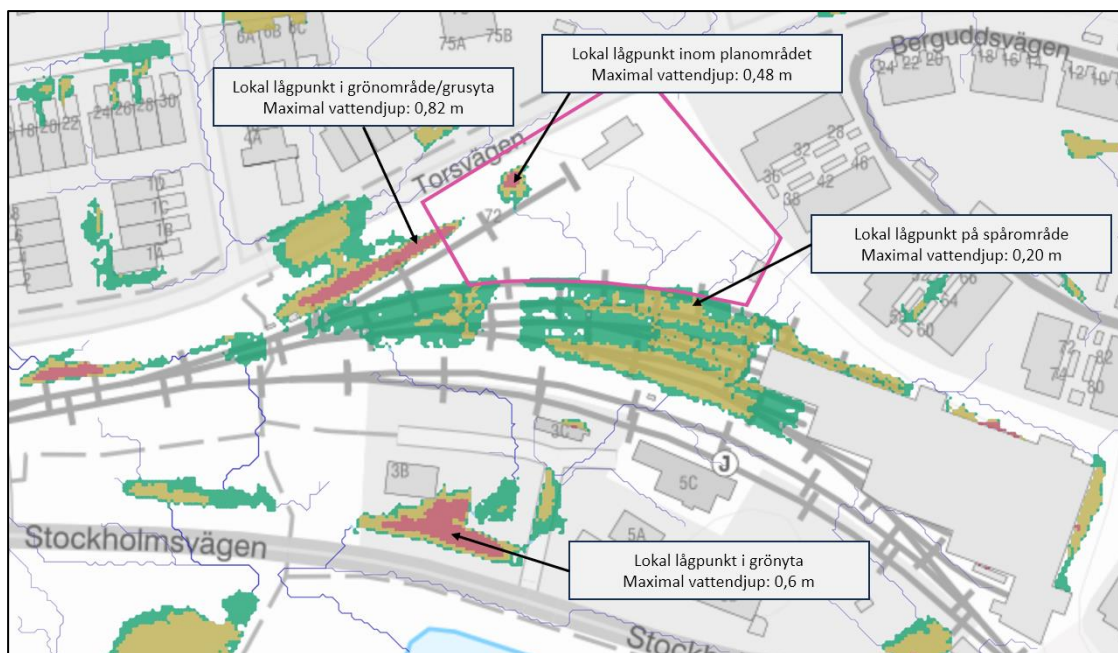
Figur 8. Översvämningsutbredning vid en nederbördsmängd på 56 mm, motsvarande ett 100-årsregn med klimatfaktor 1,25 och varaktighet 30 minuter. Maximalt vattendjup har delats in med intervallen <10 cm i grönt, 10–30 cm i gult och >30 cm i rött. Flödesvägar i mörkblå linje. Planområdet markerat med magentafärgad linje. Analysen är gjord utan funktionen "drainage".
