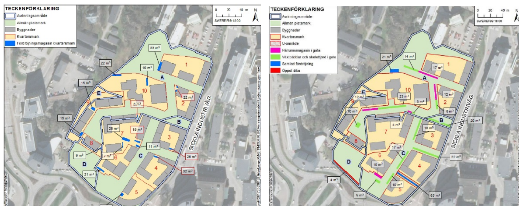
Förslag på placering av fördröjningsmagasin på kvartersmark och erforderliga magasinsvolymer samt förslag på placering av skelettkärl och hälrumsmagasin på allmän plats och erforderliga magasinsvolymer. Magasin som behöver U-områden i plankartan har markerats med röd skraffering.
