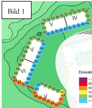
Ekvivalent ljudnivå vid fasad, högsta nivå vid någon våning, samt markering av ljuddämpad sida. Bild: Structor
