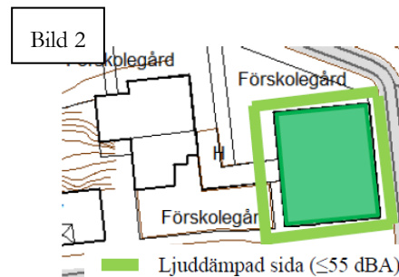
Ekvivalent ljudnivå vid fasad, högsta nivå vid någon våning, samt markering av ljuddämpad sida. Bild: Structor
